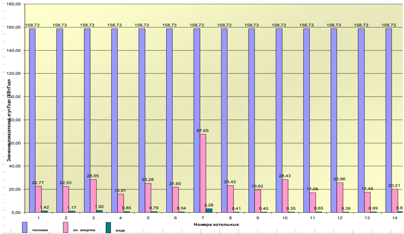
Значения удельных расходов топлива, эл. энергии и воды на выработку 1 Гкал тепловой энергии ( по котельным № 1 -- 14 )
