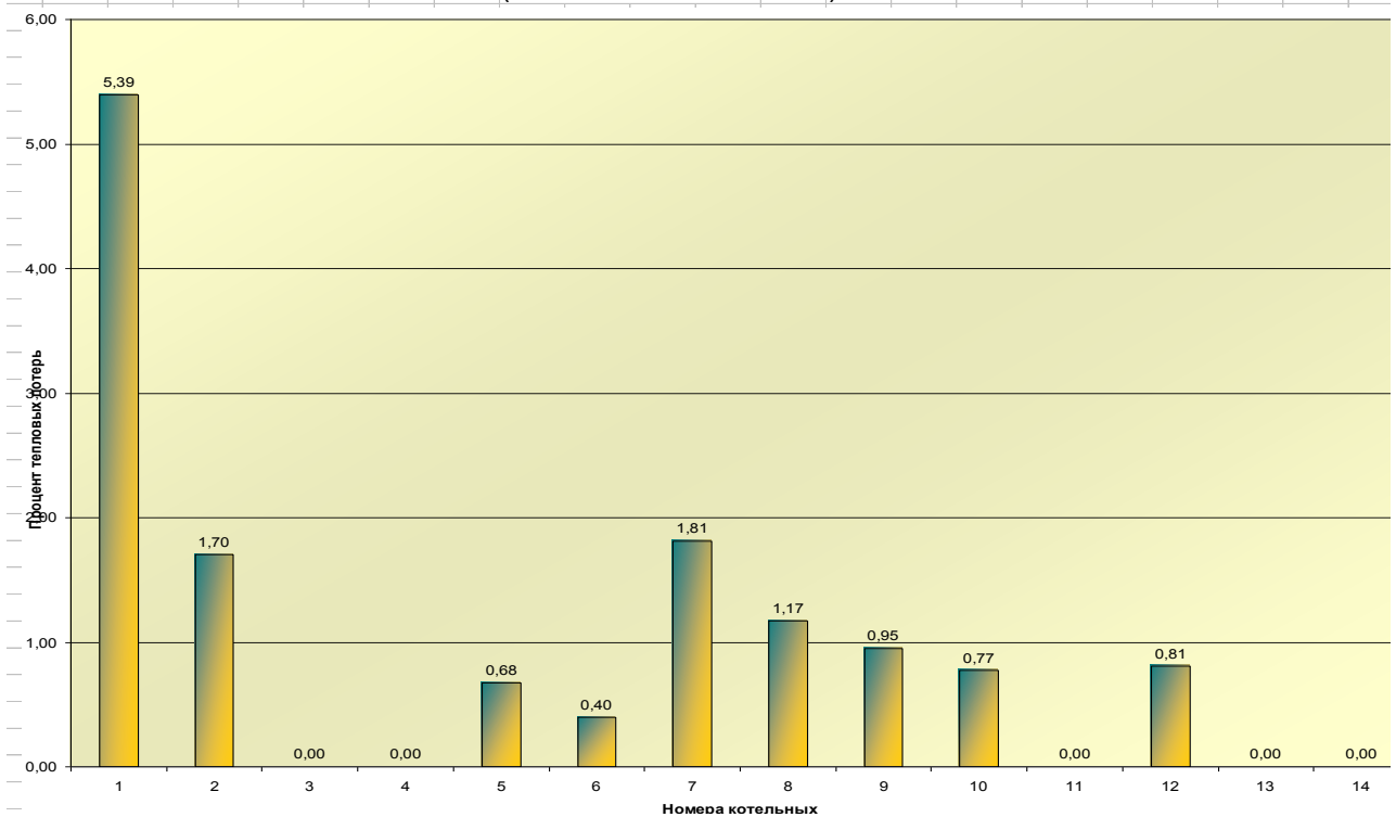
Потери ( % ) тепла через теплоизоляционную конструкцию трубопроводов теплосети ( по котельным № 14 — 14 ) Лист не печатать !
